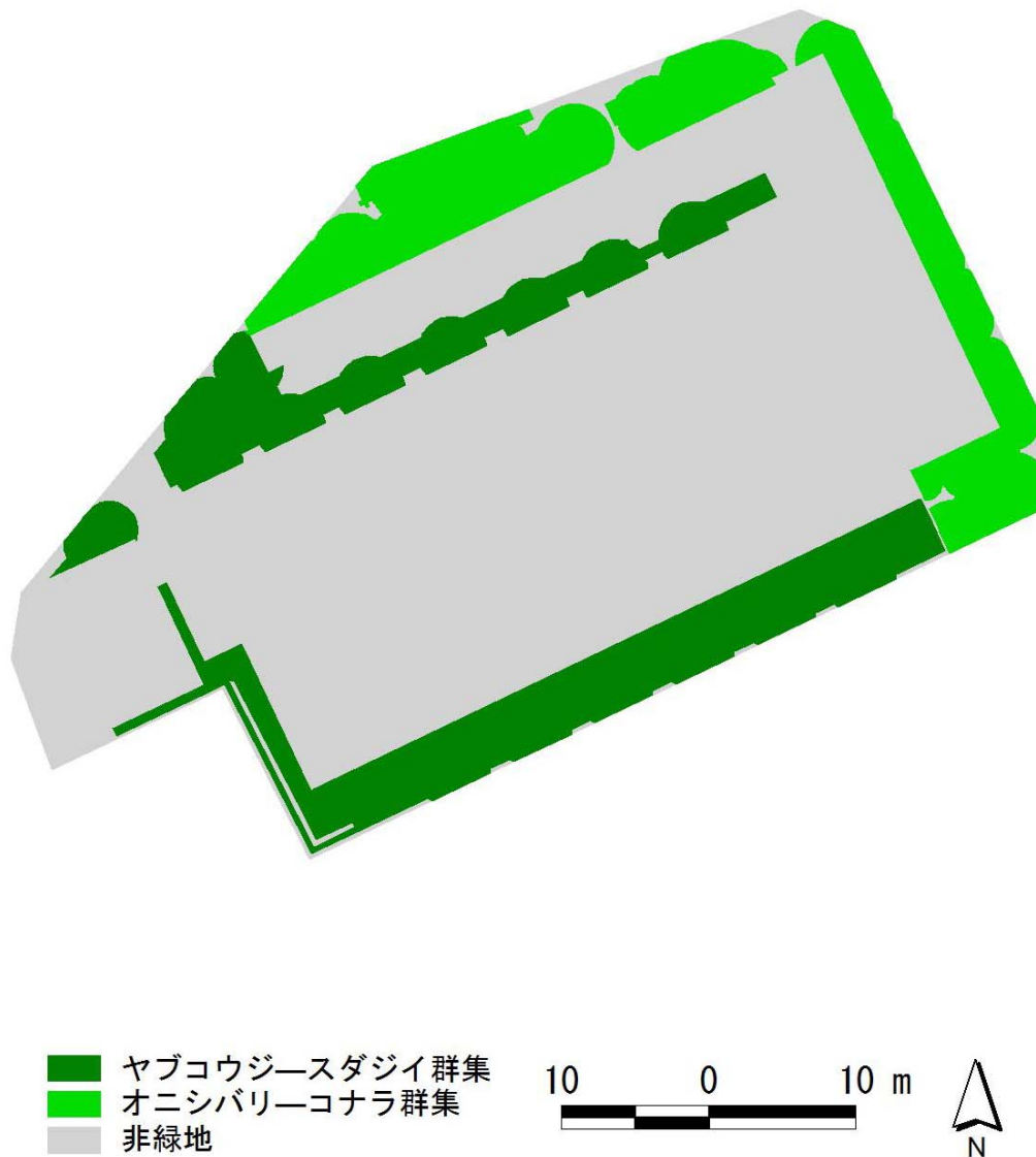
図. VEI 算出のための目標植生の配置状況
