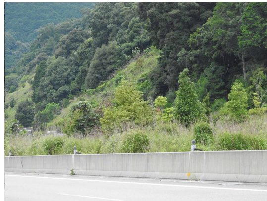
地域性苗木が植栽された中央分離帯
